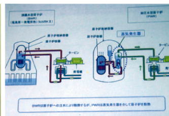
福島原子力発電所と大飯原子力発電所の 方式の違いの説明
