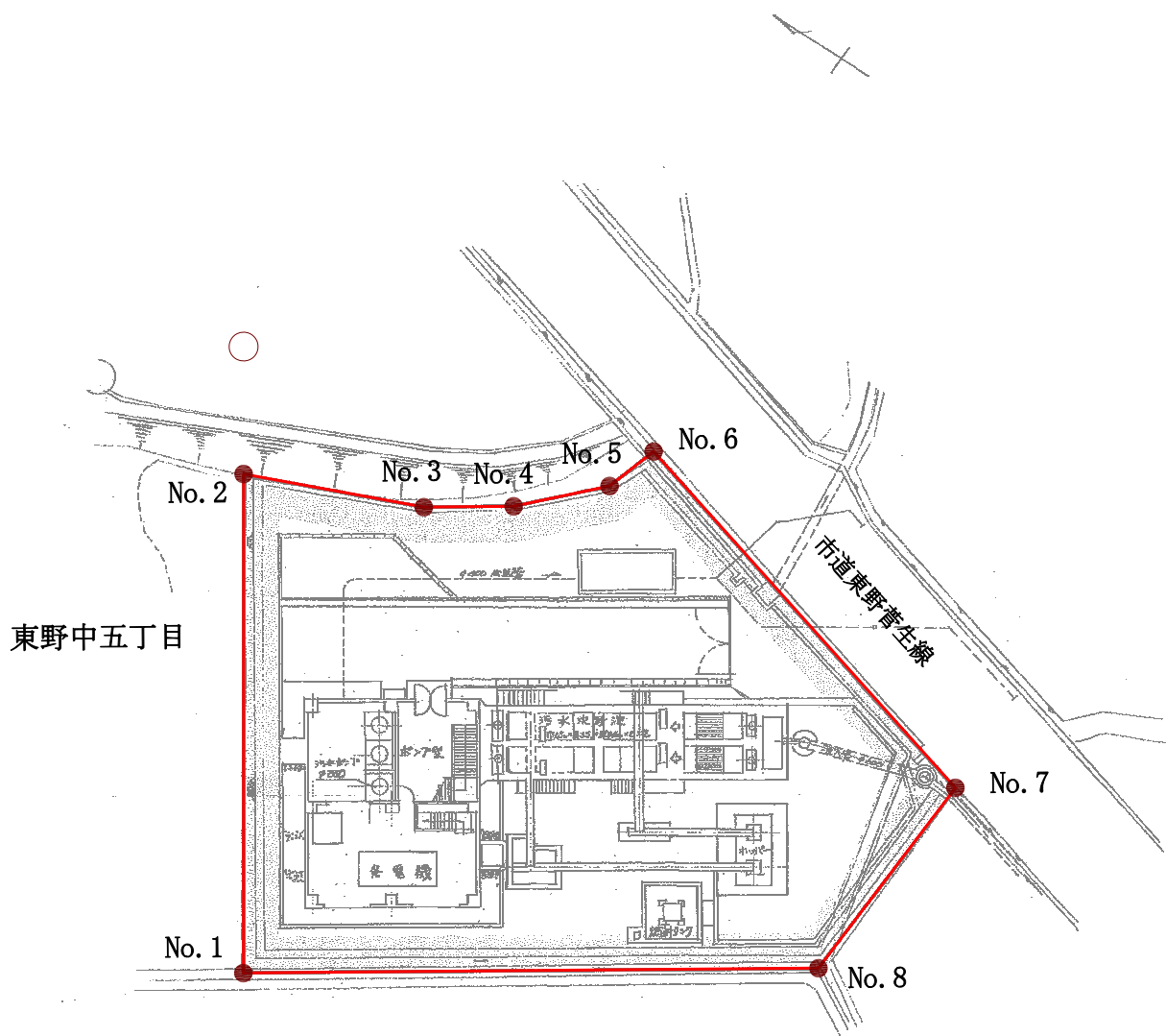
平面図 S=1/200
