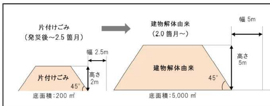
図表18 片づけごみを考慮した仮置場検討イメージ
