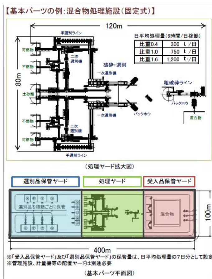
図表16 二次仮置場レイアウト図
