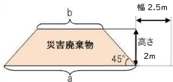
横断面図
