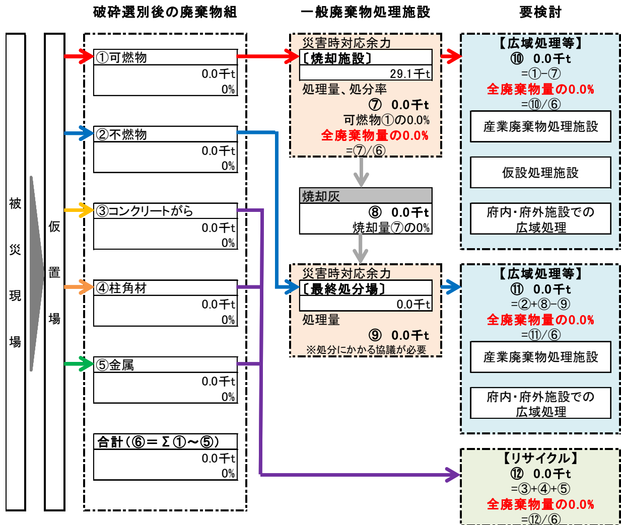
図表3-5-2 災害廃棄物処理フロー（風水害）
