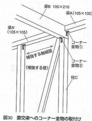
図30 直交梁へのコーナー金物の取付け
