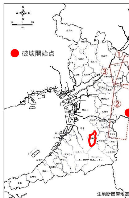
【破壊開始点】
