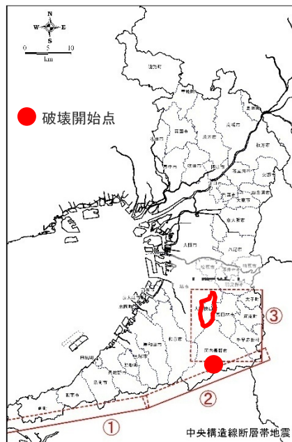
【破壊開始点】
