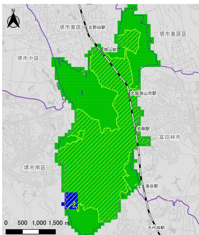
【想定地震】
