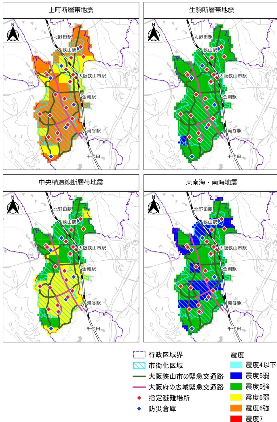
図 9-1 震度予想図
