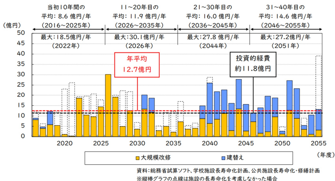
図 10-2 施設の長寿命化を考慮した場合の公共施設の更新費用等推計
