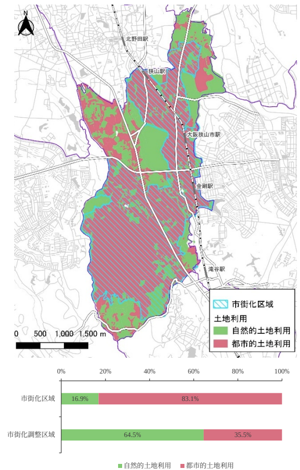
図 3-1 自然・都市土地利用図
